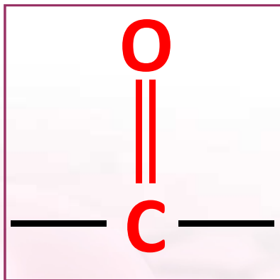
KARBONILNA GRUPA
