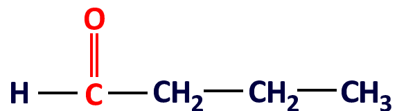
butanal
