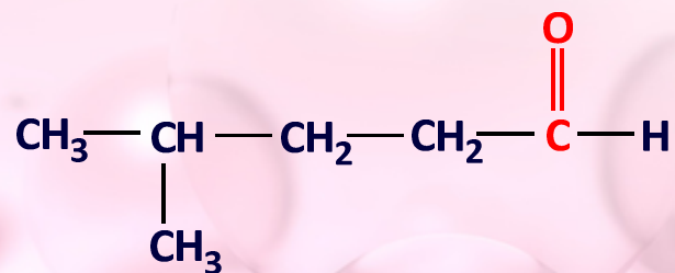
4-metil-pentalal
